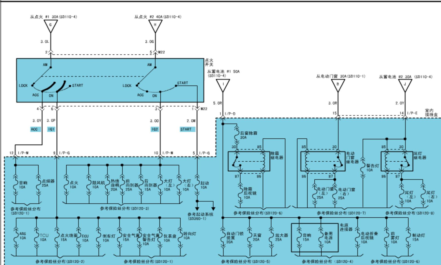
电源分布 (5)
