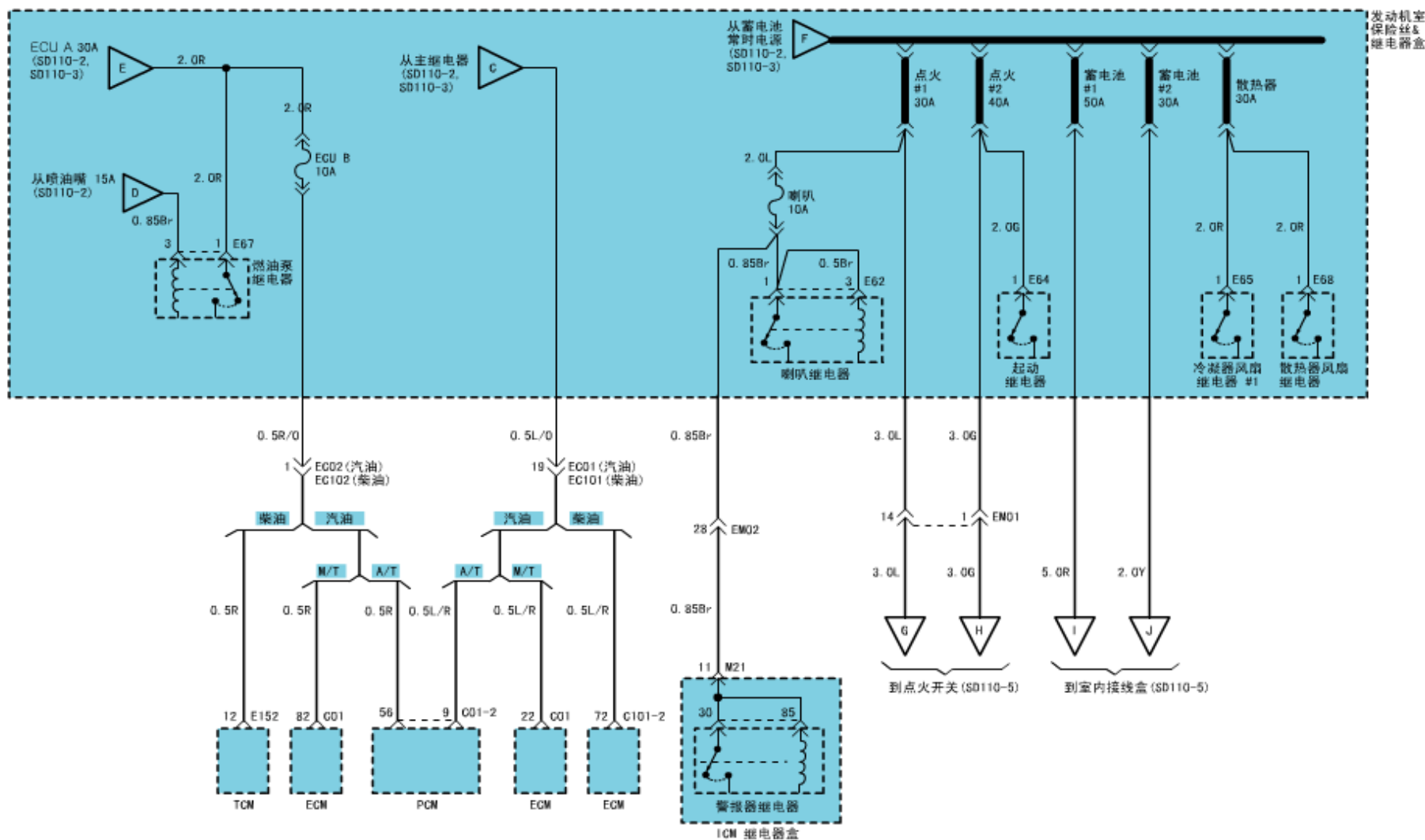
电源分布 (4)
